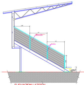
ELEVACION LATERAL DETALLE DE BARANDA
