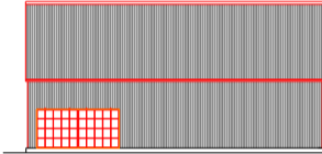
ELEVACIÓN POSTERIOR ESCALA 1:50
