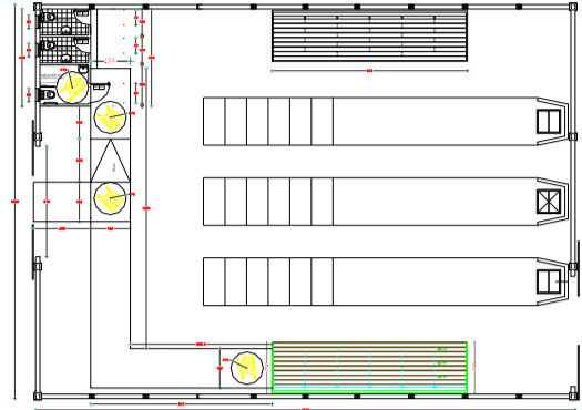
PLANTA DE ARQUITECTURA ESCALA 1:50
