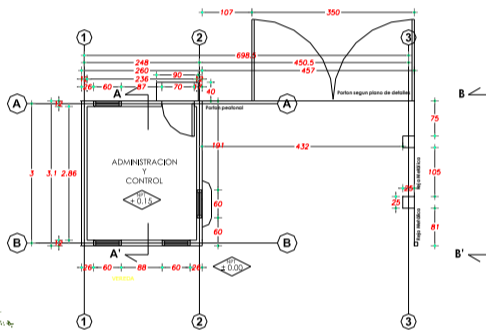
Planta General
