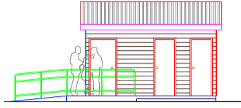
ELEVACIÓN BAÑOS ESCALA 1:50
