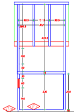
Corte A - A
