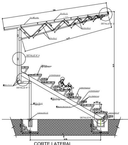
CORTE LATERAL
