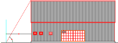
ELEVACIÓN PRINCIPAL ORIENTE ESCALA 1:50
