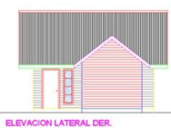
ELEVACION LATERAL DER. ESCALA 1:50
