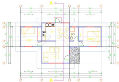
Planta General Vivienda
