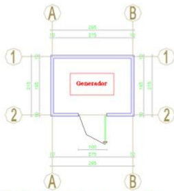
Planta Sala Generator
